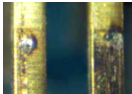
Kontaktbrand in der Anschlussstechnik – hier eine RJ45-Buchse (aus IEC 62652)
