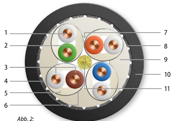
Abb. 2: Ethernet-Kabel Kat. 7
